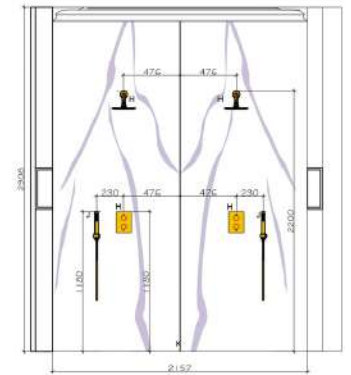
ELEVATION 6
