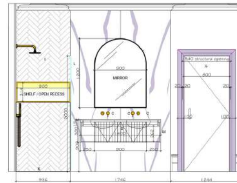
ELEVATION 4
