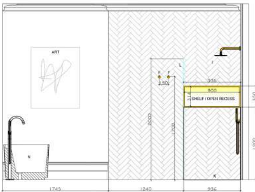
ELEVATION 2
