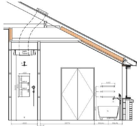
ELEVATION 1
