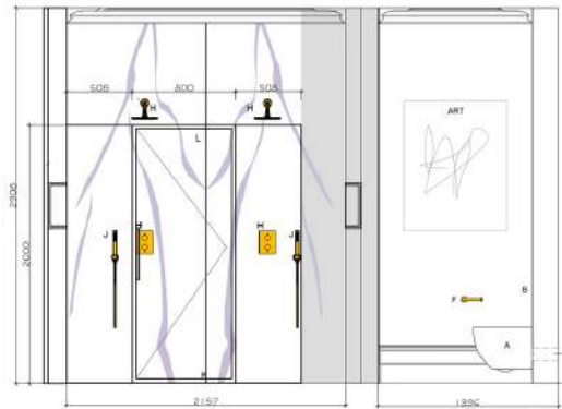
ELEVATION 3
