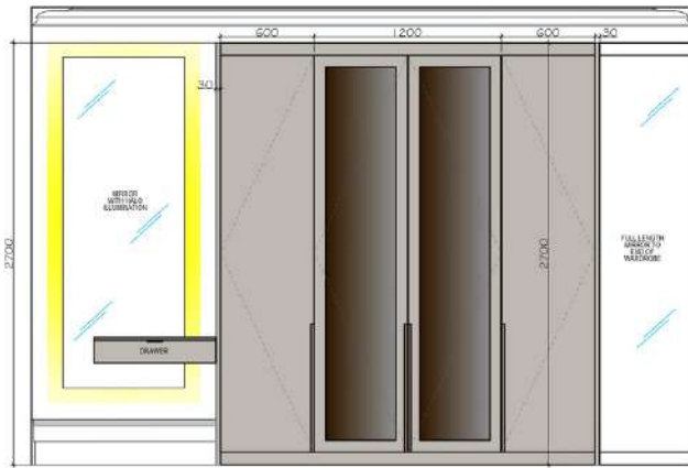
ELEVATION A
