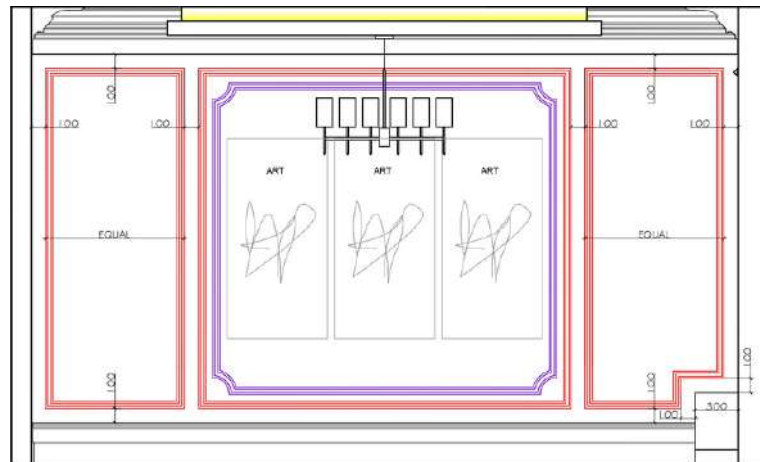
ELEVATION 4
