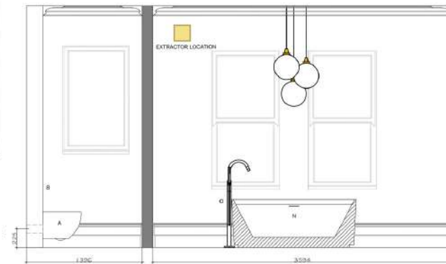
ELEVATION 1
