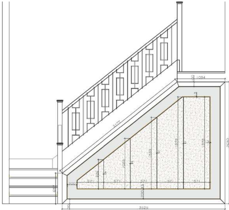
ELEVATION A
